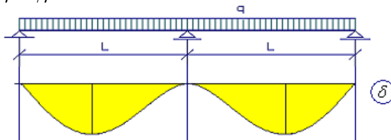
Abb. 1.5: Die Durchbiegung des Zweifeldträgers \delta
