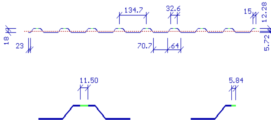
DIE DURCHSCHNITTSPARAMETER T 18 A
