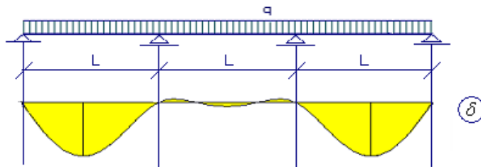
Abb. 1.6: Die Durchbiegung des Dreifeldträgers \delta
