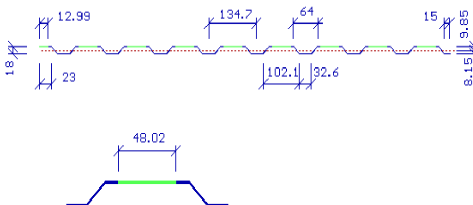
Abb. 2.3: Querschnittsform T 18 B
